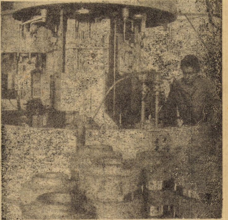
I.M.A. Sibiu. Vă prezentăm o imagine de la prelucrarea unor componente cu ajutorul unui strung, dotat cu axe verticale
