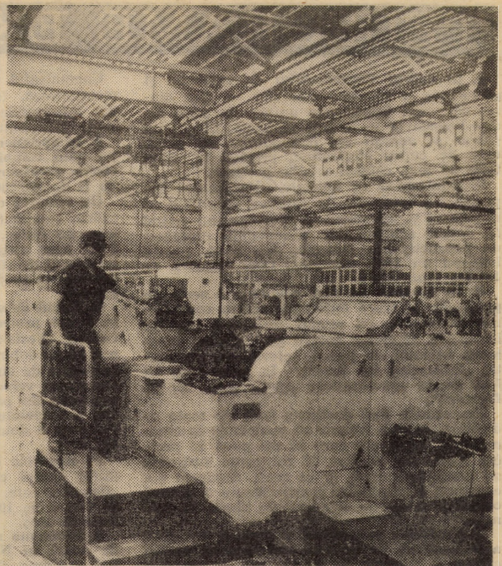
În atelierul prelucrării-presare, aparținînd secției lanțuri cu role a întreprinderii „Independența” Sibiu, la o presă multifuncțională orizontală — utilaj de mare complexitate, realizat de întreprinderea mecanică Sibiu — se realizează rolele pentru lanțurile agricole și cele destinate industriei petroliere. Noul utilaj de mare productivitate, alimentat prin material livrat în colaci, execută rolele la cote finite fără a necesita prelucrări ulterioare. Foto: Fred NUSS
