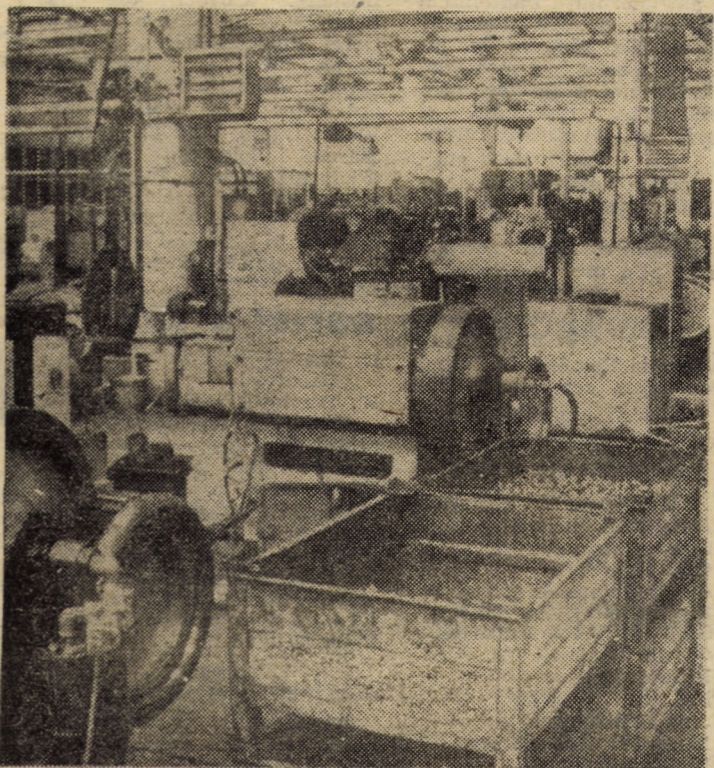
Vedere de ansamblu din interiorul secției lanț cu role, a întreprinderii „Independența” Sibiu. În prim-plan — mașini automate de rulat și calibrat-bucși, utilaje de înalt randament. Foto: Fred NUSS
