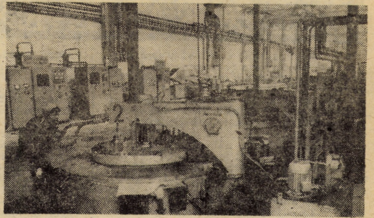
Vă prezentăm o vedere parțială a atelierului tratamente termice din secția lanț cu role a întreprinderii „Independența” Sibiu
