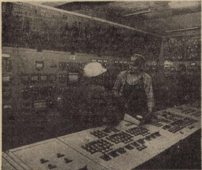
I.M.M.N. Copșa Mică. Executarea comenzilor, precum și urmărirea parametrilor funcionali ai furnalului, sînt efectuate din camera de comandă
