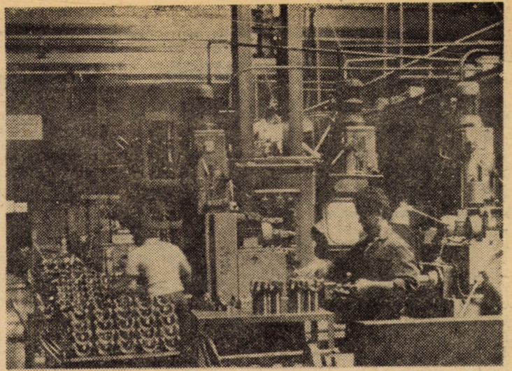
Întreprinderea de piese auto Sibiu: aspect din secția transmisii cardanice, unde operațiunile de prelucrare și asamblare se execută cu dispozitive ce asigură parametrii calitativi prevăzuți în documentațiile tehnice Foto: Fred NUSS
