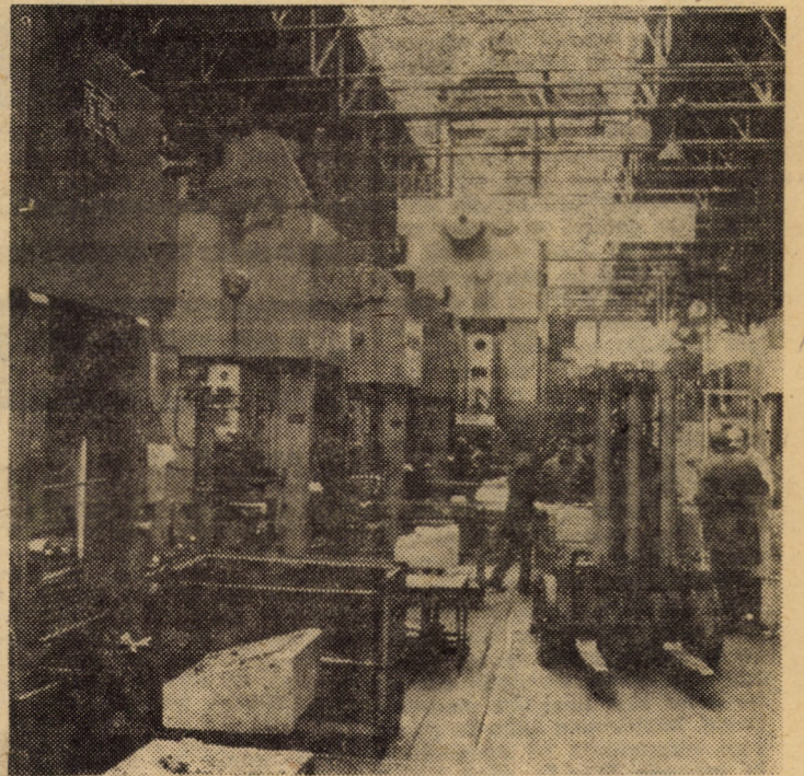
Vedere din secția prelucrării mecanice a întreprinderii „Emailul roșu” Mediaș. În prim-plan: grupul de prese cu transfer
