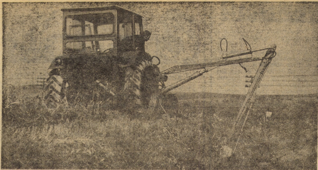
O noutate in activitatea de intretinere a lucrarilor de imbunatatiri funciare din cadrul I.E.E.L.I.F. Sibiu: dotarea sectoarelor cu echipamente de curatit canale (E.C.C.) montate pe tractoare U-650. In imagine: mecanizatorul Alexandru Dorca executa decolmatarea unui canal din sistemul de desecare Avrig - Scorei Foto: ing. Mircea COLCERIU
