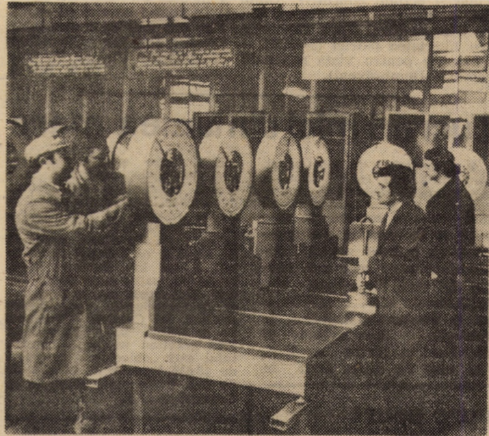
Întreprinderea „Balanța” Sibiu — probe metrologice la balanțe semiautomate de 100 kg.
