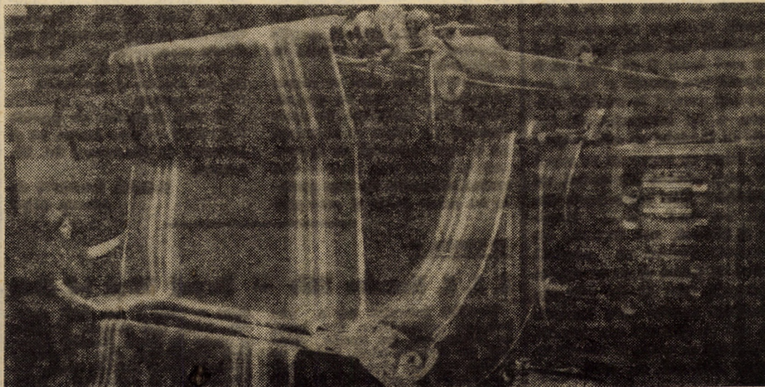
Întreprinderea textilă „Dumbrava” Sibiu. Înainte ca păturile „Tufted” și cuverturile să ajungă în fazele croit și finisat, acestea parcurg operația de scămășat, operație efectuată cu ajutorul unui utilaj de mare randament, pe care vi-l prezentăm în imagine Foto: Fred NUSS
