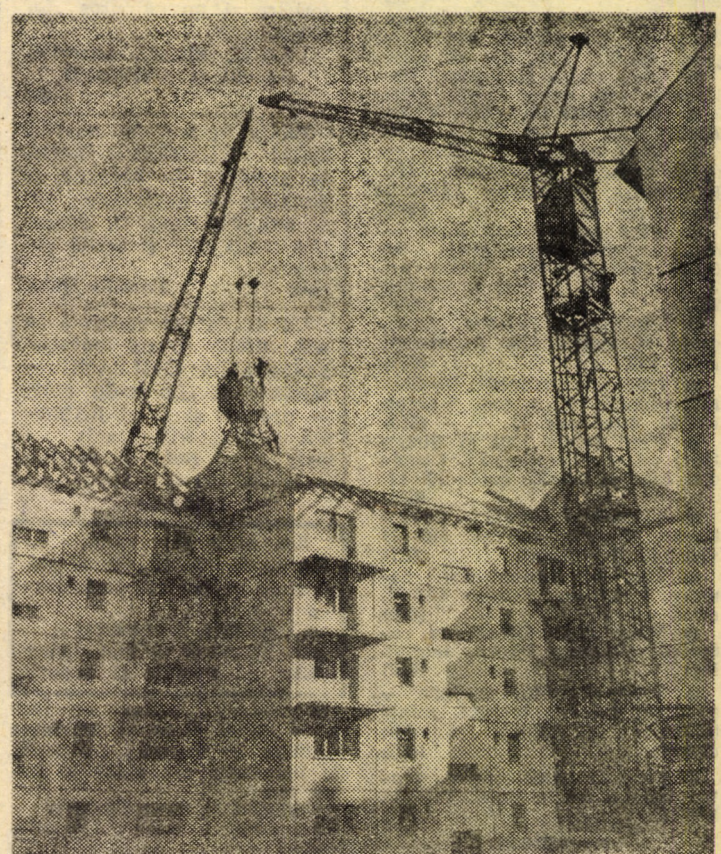
Suita blocurilor de locuințe ridicate pe str. Rusciorului din Sibiu completează armonios peisajul arhitectonic al tînrului cartier „11 Iunie” din zona industrială a „orașului de jos”. În fotografie: lucrări la șarpanta învelitoare a blocului 71, executate de echipele conduse de Gheorghe Olteanu și Mihai Weber din brigada complexă nr. 2 a I.A.C.M. Sibiu.
