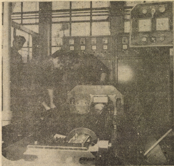
Vă prezentăm în imagine pe lăcătușii Ioan Borcea și Ilie Crețu din secția sculară a Întreprinderii „Mecanica” Sibiu lucrînd la un nou tip de extruder pentru mase plastice, aflat în fază de probe tehnologice Foto: Fred NUSS
