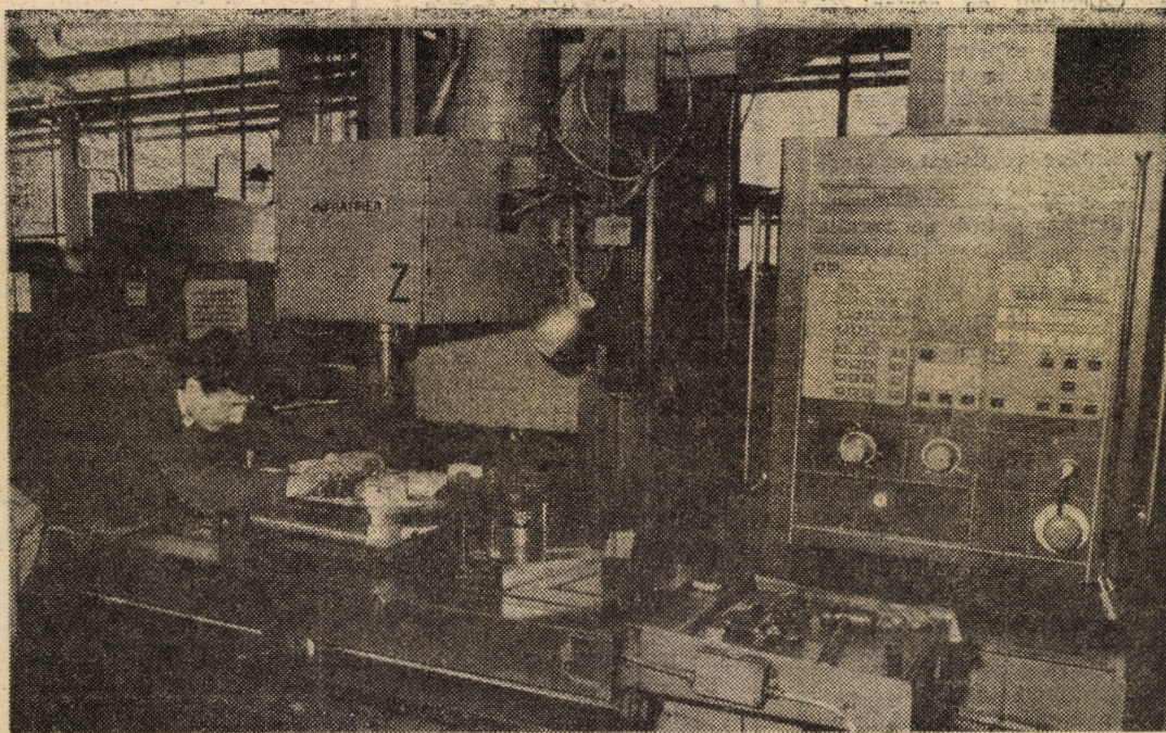
La o freză verticală cu comandă numerică, recent intrată în dotarea secției scolare a Întreprinderii „Mecanica” Sibiu, se prelucurează piese de complexitate ridicată și cu înaltă precizie
