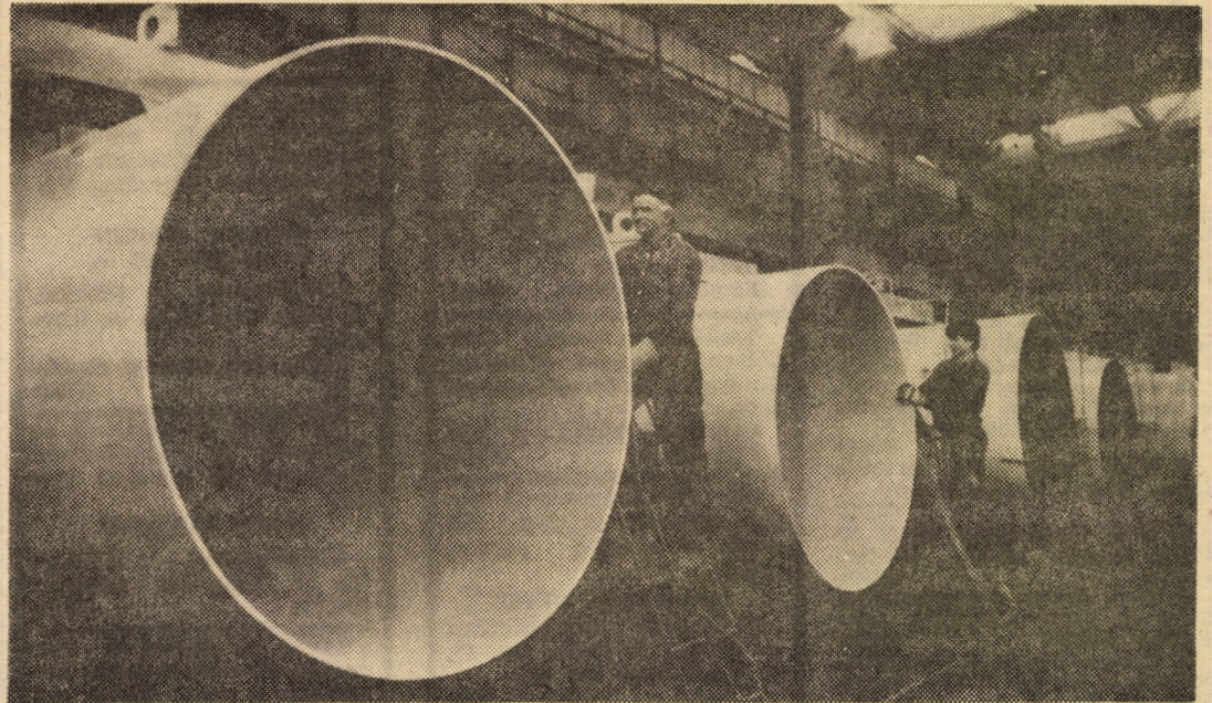
Întreprinderea „Independenţa” Sibiu. Elemente componente din conducta forţată destinată exportului, aflate în fază de vopsit-finisaj Foto: Fred NUSS
