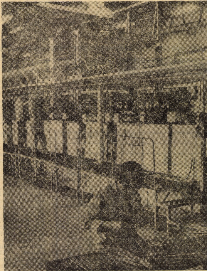
I.P.A. Sibiu. Vedere parțială a liniei de cromare dură pentru tije amortizoare telescopice, instalație de înaltă productivitate
