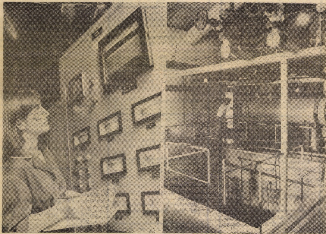
Întreprinderea „Furul Roșu“ Tâlmăciu dispune de o modernă stație pilot cu ajutorul căreia se recuperează soda caustică din apele reziduale. În stînga, Elena Halmagiu, operator chimist, în fața tabloului de comandă al instalației, urmîrind parametrii de funcționare ai stației
