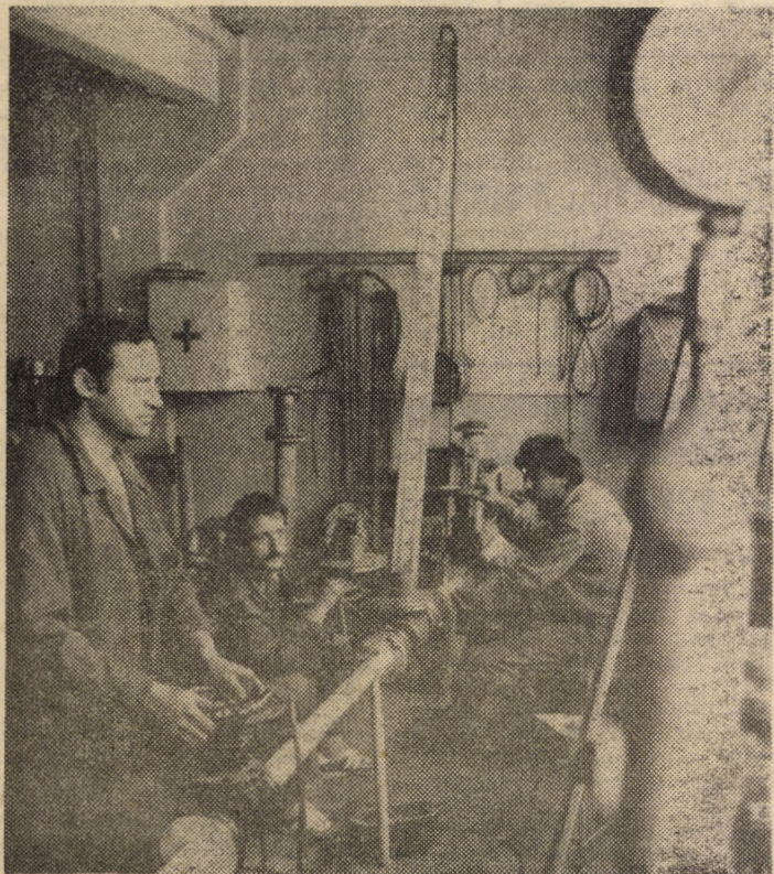
Întreprinderea Mecanică pentru Gaz Metan Mediaș. În imagine — standul de probe pentru aparatură pneumatică
