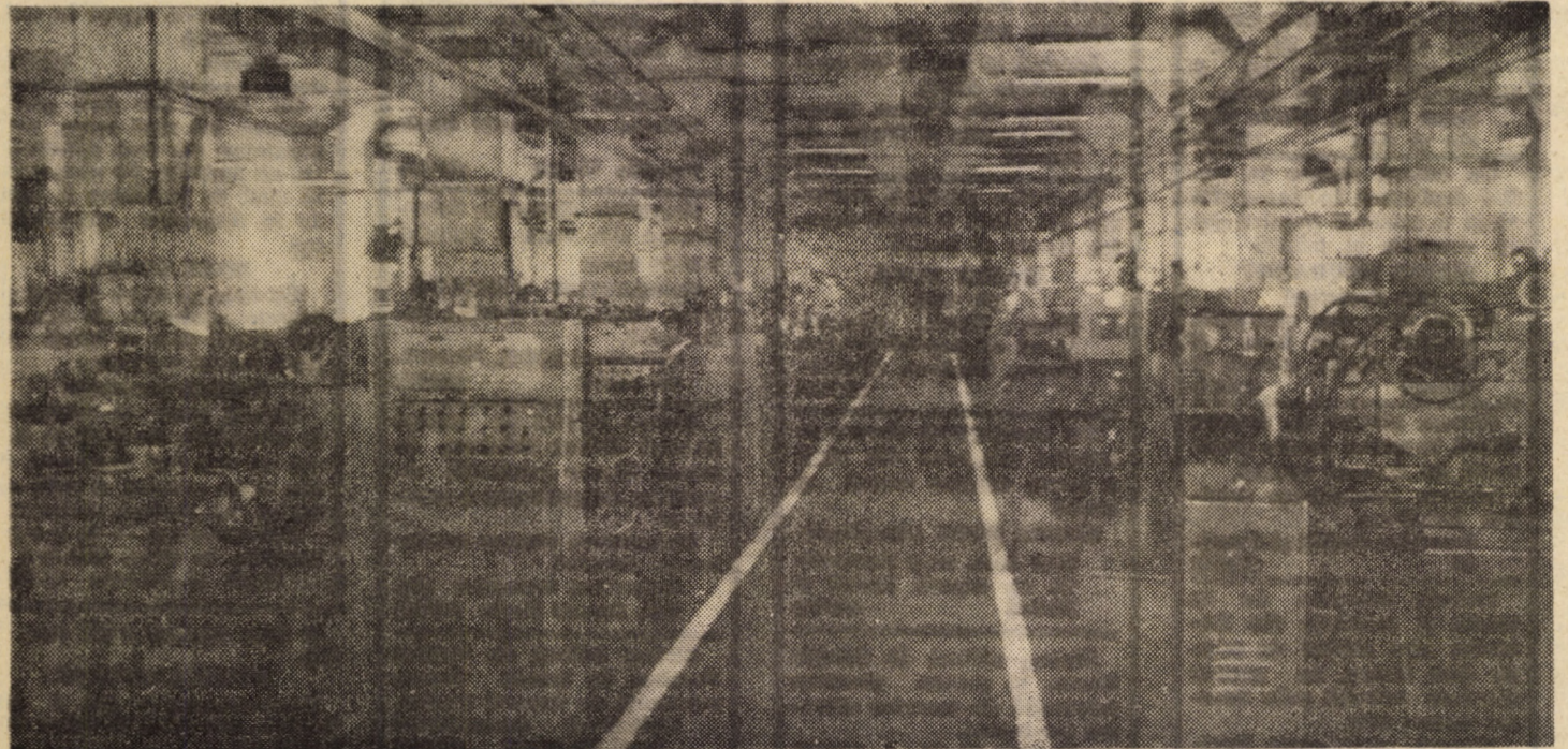
Vedere de ansamblu a halei de unelte pneumatice de la Întreprinderea „Independența” Sibiu
