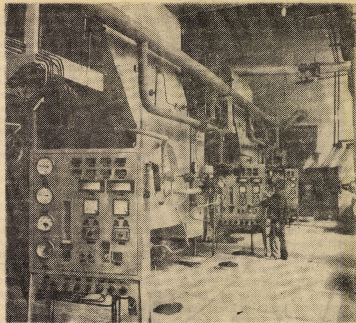
Vă redăm o imagine dintr-o modernă centrală termică, aparținînd Întreprinderii „Furul Roșu” Tălmăciu, care facilitează bunul mers al procesului tehnologic din sectorul finisaj umed Foto: Fred NUSS
