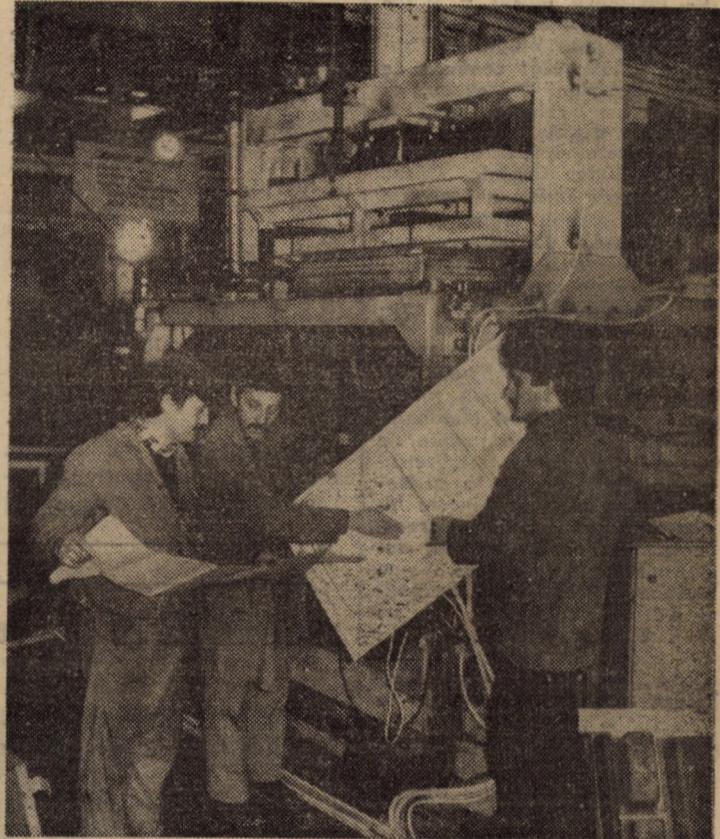
Intreprinderea Mecanica Sibiu. Printre realizările de ultimă oră ale prestigioasei unități constructoare de mașini se înscrie și agregatul pentru termoformare mase plastice de tipul ATF-4, destinat exportului. În fotografie: ing. Dumitru Capotă, proiectant principal, lăcătușul Ilie Cojocaru și reglorul Lucian Istrătescu urmărind calitatea primelor produse obținute Foto: Fred NUSS
