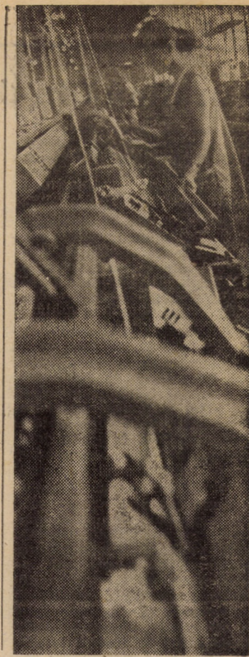
Întreprinderea „Drapelul Roșu” Sibiu. La noile mașini rectilini de tricotat R 50, de producție românească se realizează în prezent o gamă variată de tricotate tip jacard, destinată beneficiarilor externi Foto: Fred NUSS
