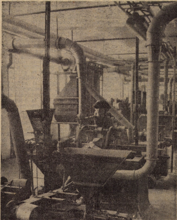
Linie modernă de prelucrare a scindurelelor din noua capacitate de producție a Fabricii de creioane a I.P.L. Sibiu Foto: Fred NUSS
