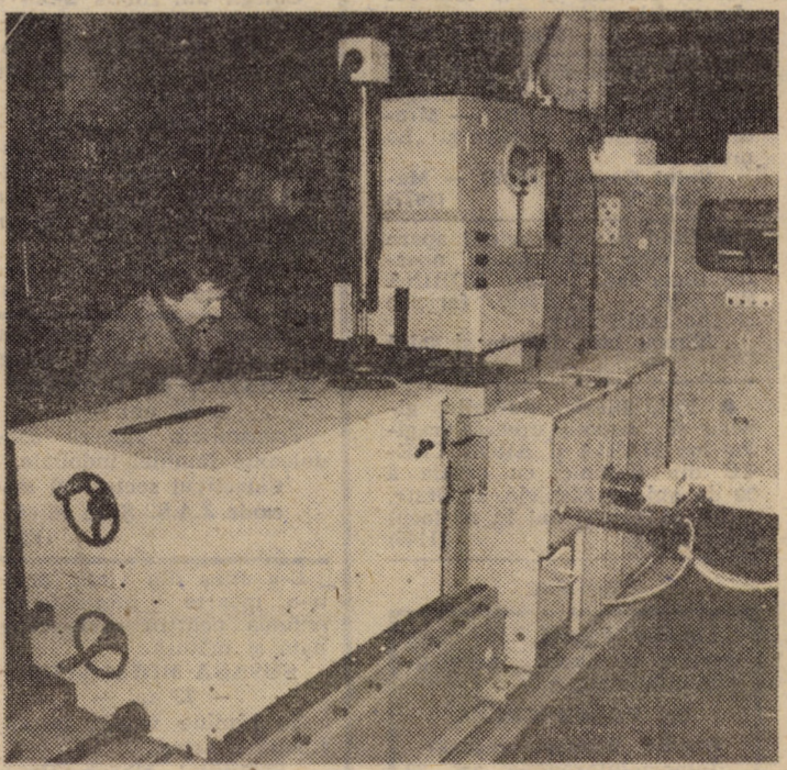
Printre noile realizări ale constructorilor de utilaje de la Întreprinderea Mecanică Sibiu figurează și mașina de ansoșat în pași, destinată industriei electrotehnice, pe care v-o prezentăm în fotografia de față Foto: Fred NUSS
