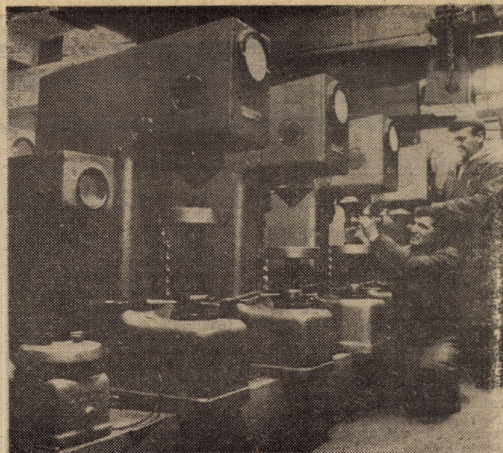
În secția II lăcătușărie-montaj a întreprinderii „Balanța” din Sibiu, șeful de echipă Andrei Hartmann și lăcătușul Constantin Foamele pregătesc un nou lot de aparate pentru încercat duritatea metalelor prin metoda „Brinell”, urmînd a fi livrate beneficiarilor interni și externi Foto: Fred NUSS
