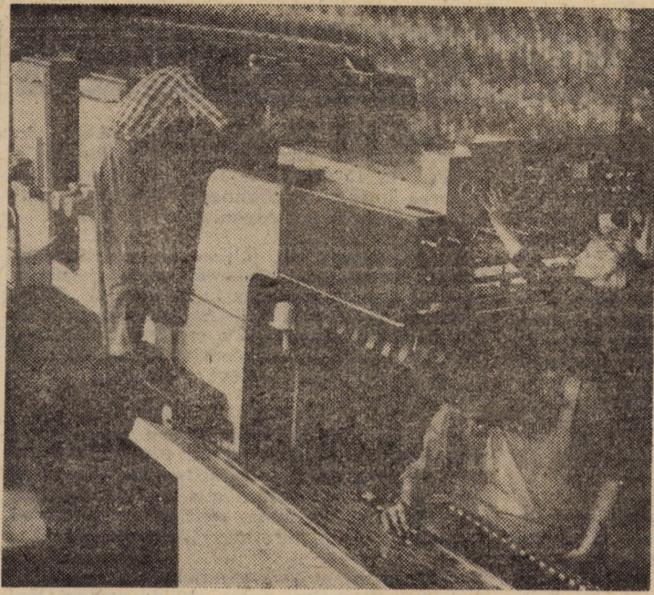
Printre unitățile economice din județul nostru, cu bune rezultate în întrecerea socialistă, se află și Întreprinderea Poligrafică Sibiu. În imagine, aspect de muncă din secția Ofset, la unul din modernele utilaje — mașina de tipărit în cinci culori Foto: Horst BUCHFELNER
