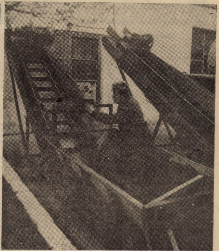
Incărcătorul de știuleți pentru batoza de porumb BP-15, cu o capacitate de 15 tone/oră — produs realizat de I.M.A. Sibiu
