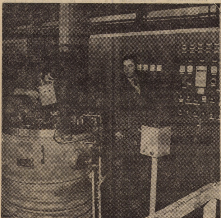
Întreprinderea Mecanica Sibiu: instalație de nitrurare ionică cu ajutorul căreia se aplică unul dintre cele mai avansate procedee de tratament termic pentru durificarea metalului Foto: Fred NUSS
