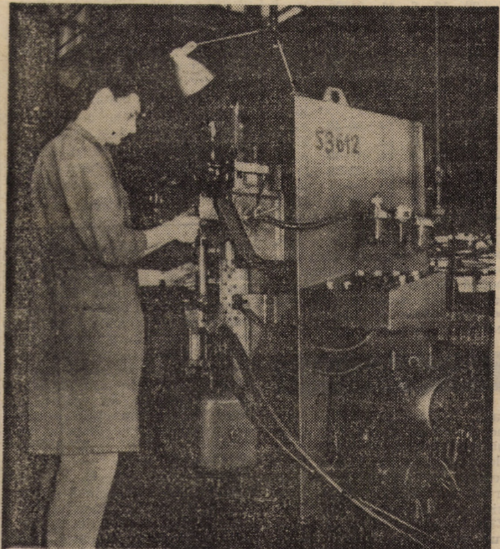
Stand pentru verificarea diagramei a amortizoarelor pentru autoturisme — unul dintre utilajele realizate prin autoutilare din secția amortizoare hidraulice de la I.P.A. Sibiu
