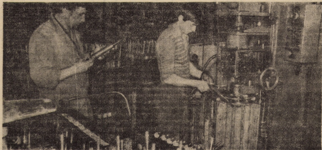
Operațiunea de sertizare a amortizoarelor în secția amortizoare hidraulice de la I.P.A. Sibiu Foto: Fred NUSS
