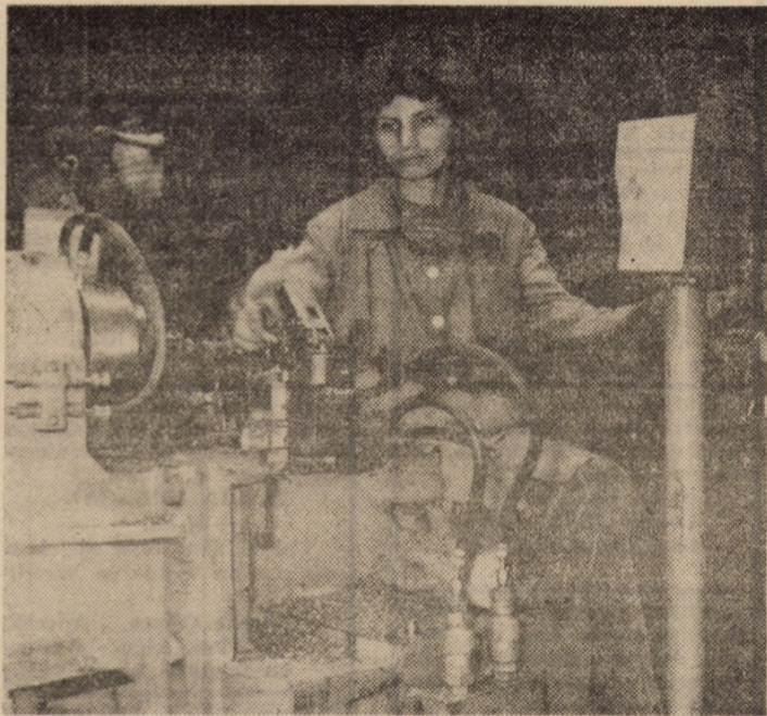
I.P.A. Sibiu, secția servo-direcții hidraulice. La un utilaj, realizat prin autoutilare, se execută frezarea furcii cu gît a axului volan pentru autoturismele Olteit Foto: Fred NUSS
