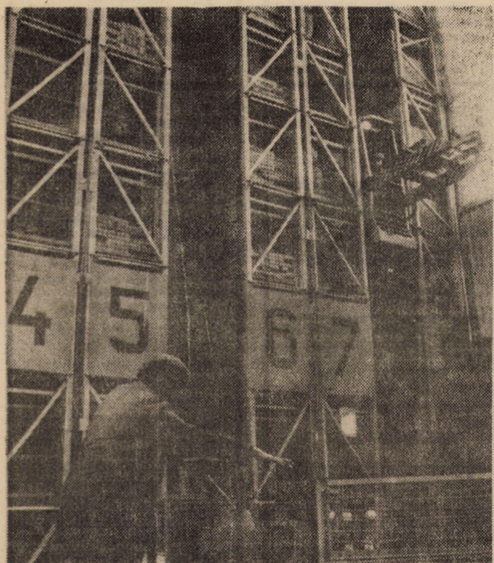
Imagine parțială a depozitului pe verticală cu gestiune automată pentru materiale semifabricate, S.D.V.-uri etc, recent dat în folosință la I.M.A. Sibiu Foto: Fred NUSS
