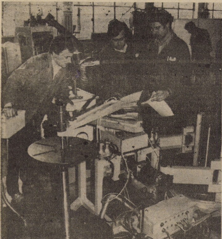
În secția sculară a Întreprinderii Mecanica Sibiu se află în curs de finalizare un utilaj complex, alcătuit dintr-o mașină de ancrasat în pași de 6 t/f și un dispozitiv de alimentare, care va fi prezentat la „T.I.B. '89” din toamna acestui an. În fotografie: maestrul Nicolae Dordea (mijloc) împreună cu lăcătușii Ion Borcea și Ion Poponea pregătind noul utilaj pentru probe tehnologice. Foto: Fred NUSS
