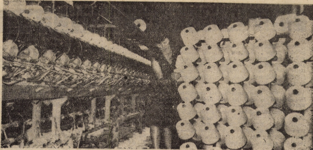
Faza de rebobinare a firelor de bumbac la o mașină „IMATEX”, utilaj de mare productivitate din secția bobinat a Întreprinderii „7 Noiembrie” Sibiu. Foto: Fred NUSS
