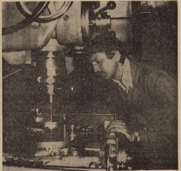
Executarea unor repere de înaltă precizie la o mașină de găurit prin coordonate în cadrul atelierului scularie al Întreprinderii Mecanica Sibiu Foto: Fred NUSS
