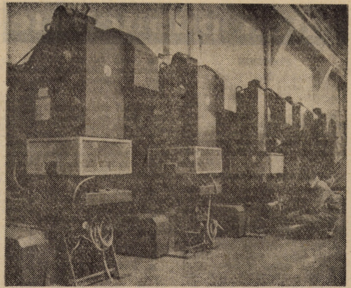
Întreprinderea Mecanică Sibiu. O ultimă verificare înainte de expediere la un lot de prese mecanice de 16 tone-forță destinat industriei constructoare de mașini Foto: Fred NUSS
