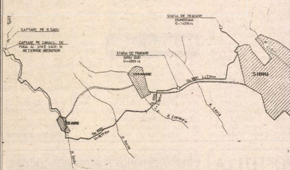
PLANUL GENERAL AL SISTEMULUI DE ALIMENTARE CU APA A MUNICIPIULUI SIBIU - Sursa Sadu -
