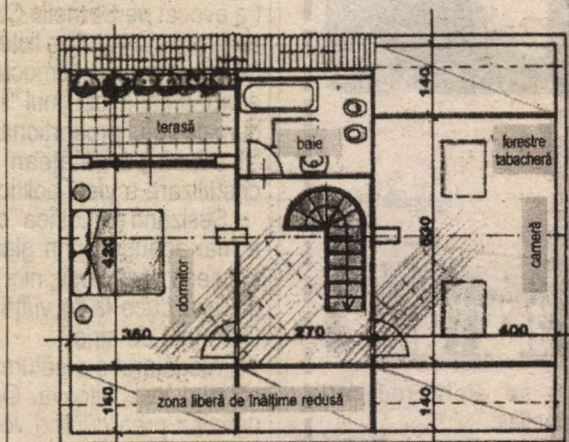
PLAN NIVEL MANSARDĂ, ÎN CARE ESTE EVIDENȚIATĂ TERASA, CELE DOUĂ DORMITOARE, BAIA, PRECUM ȘI SCARA DE ACCES
