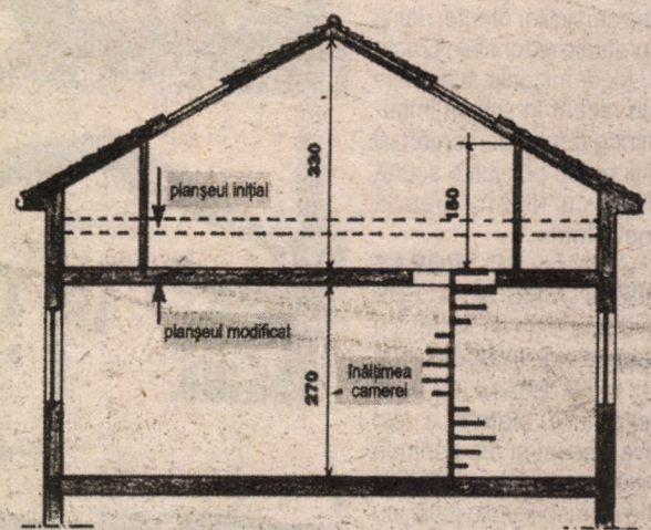
SECȚIUNE ÎN CARE ESTE PREZENTĂ SCARA DE ACCES ȘI SPAȚIUL DE PE CONȚUR, CARE RĂMÂNE NEUTILIZAT
