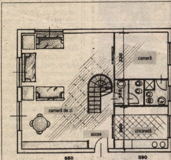
PLAN NIVEL INFERIOR, ÎN CARE SE EVIDENȚIAZĂ NOUL MOD DE ORGANIZARE A SPAȚIULUI
