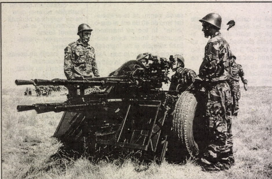
Mitraliera antiaeriană MR4, gata de tragere
